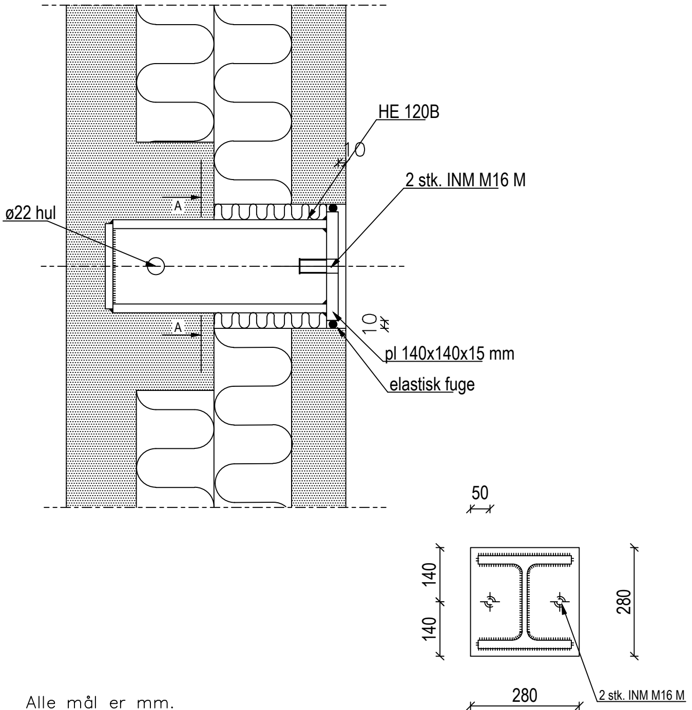
Snit A-A
