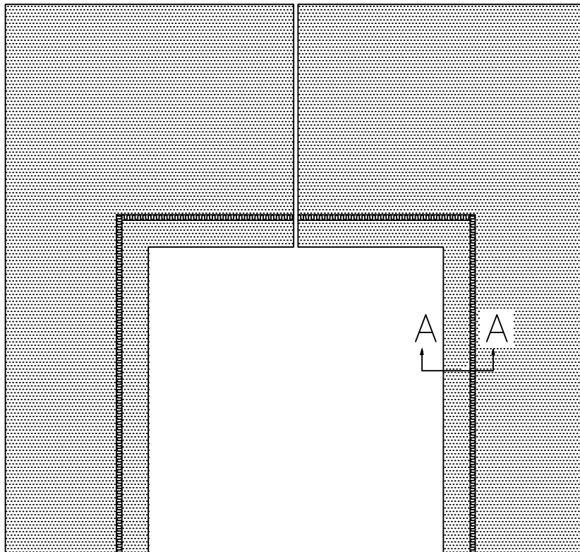
Opstalt 1:20
