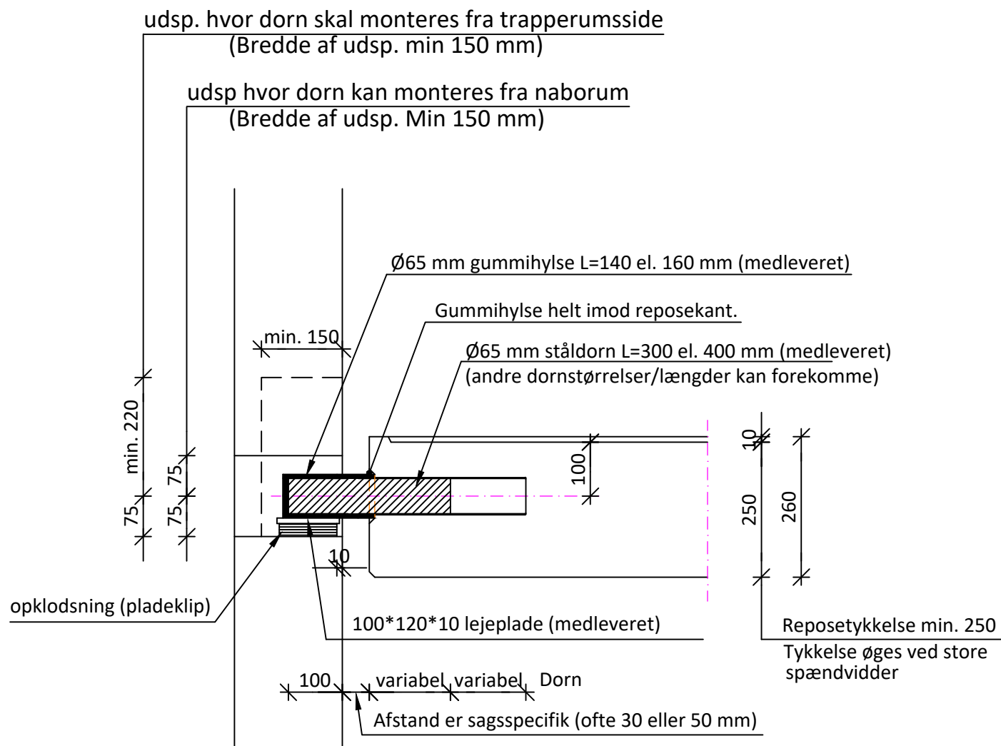
PRINCIPDETALJE VED DORN
