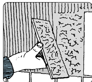
4. Kontrollér mørteldækningen. Fliseres bagside skal være dækket.
