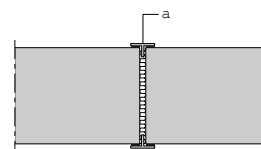
DETALJE 6
