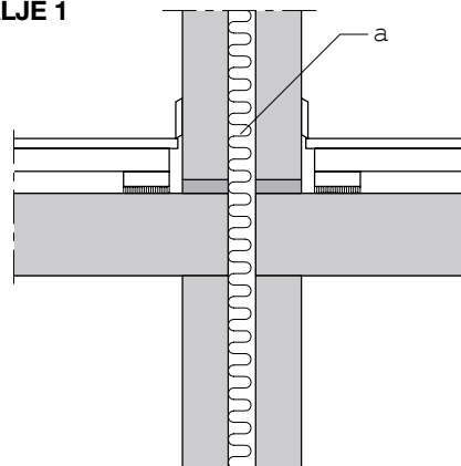
DETALJE 1
