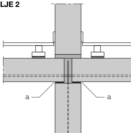
DETALJE 2
